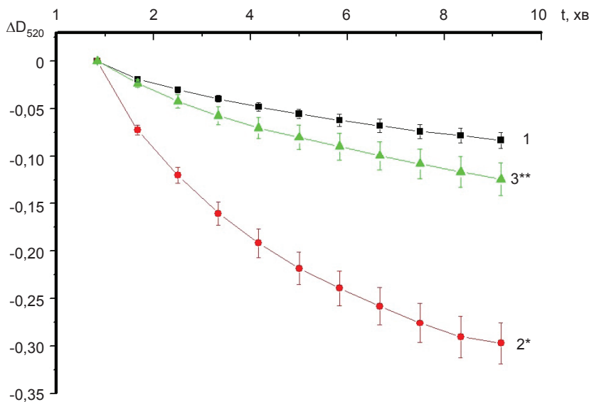
Рис. 2. Часова залежність світлопоглинання суспензії мітохондрій, виділених з сердець тварин: 1 – контроль; 2 – щури з ізопротереноліндукованим пошкодженням міокарда; 3 – з ізопротереноліндукованим пошкодженням міокарда за впливу ω-3 ПНЖК. *P<0,05 порівняно з контрольною групою, ** – порівняно з II групою
