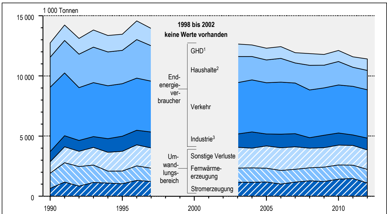
Grafik: Energiebedingte CO 2 -Emissionen aus dem Primärenergieverbrauch in Hamburg 1990 - 2012
