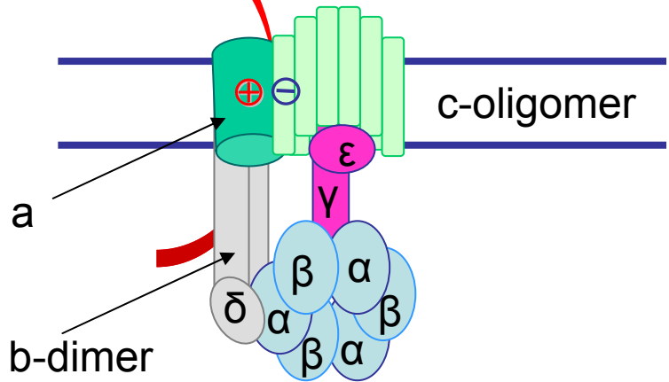
F-type ATPase
