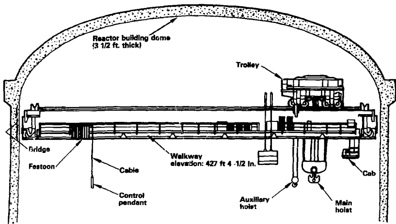
POLAR (OVERHEAD) CRANE
