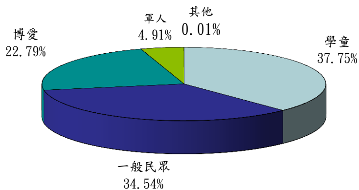
圖 5-5-4-3 乘客結構圖
