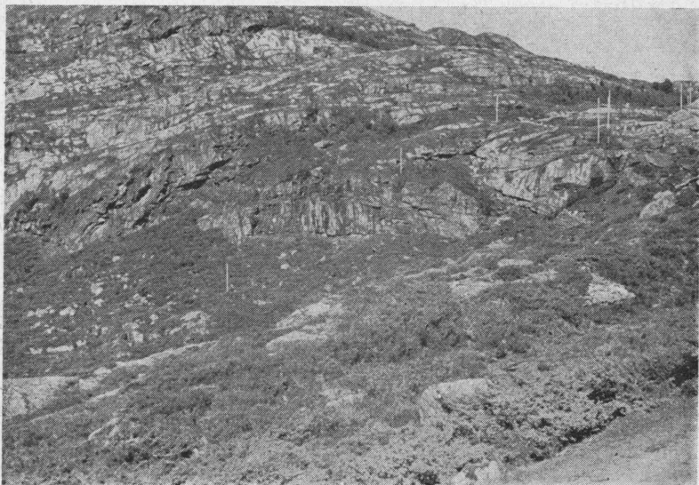
Fig. 12. Stor antiklinal ved Remme, Brattvåg. (The great anticline at Remme, Brattvåg.) T. Gjelsvik.
