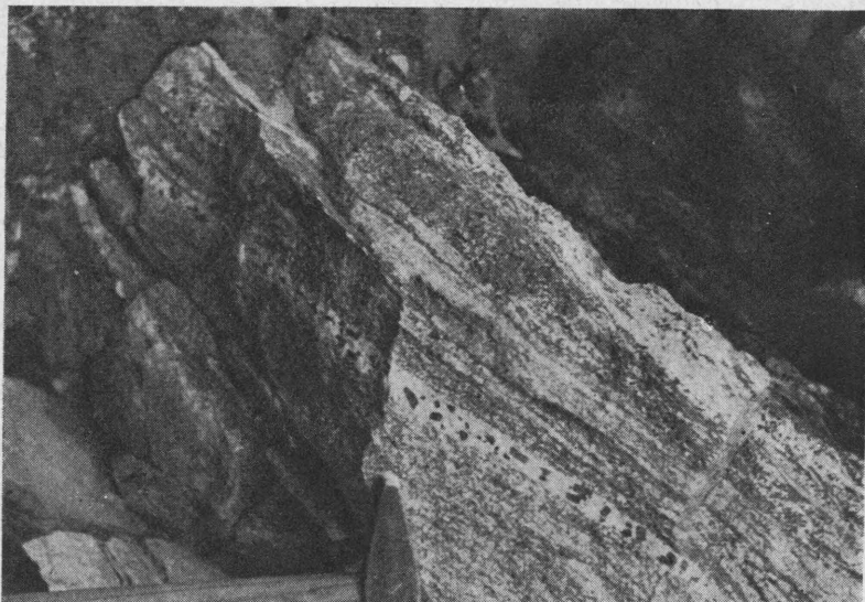
Fig. 1. Lys åre med porphyroblastisk hornblende. (Porphyroblasts of amphibole in granitic veins.) Engesetskaret, Hareidlandet. Chr. C. Gleditsch.
