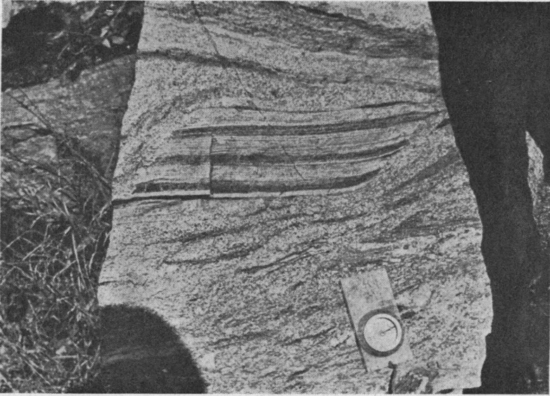
Fig. 7. Inneslutning av finkornet, finbåndet gneiss i grovkornet gneiss. (Finegrained, banded gneiss enclosed in coarse, granitic gneiss.) Dyrkorn. T. Gjelsvik.
