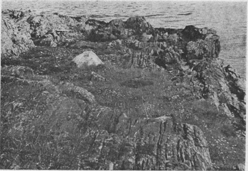
Fig. 10. Grønnskifer. (Green schist.) Hildre Brygge, Haram. T. Gjelsvik.
