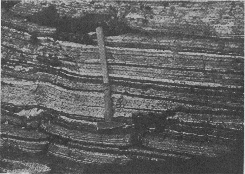
Fig. 8. Konkordante årer av grovkornet granittisk sammensetning i finbåndet gneis, av samme karakter som inneslutningen i fig. 7. De førstnevnte representert av de bredeste og lyseste bånd. (Broad, white coarsegrained veins injected into a finegrained banded gneiss, like the inclusions in Fig. 7.) Bremanger, Nordfjord. T. Gjelsvik.
