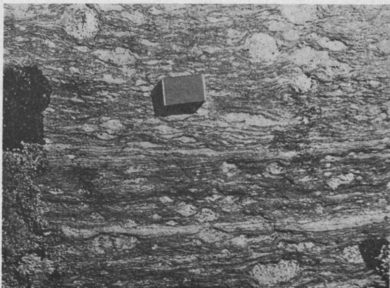
Fig. 4. Øyegneis. (Augengneiss.) Brattvåg. T. Gjelsvik.
