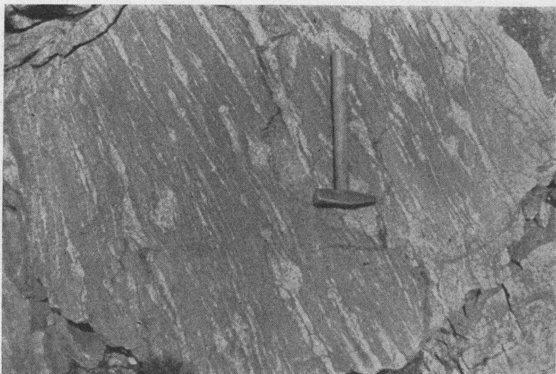
Fig. 6. Øyegneis på overgang til åregneis. (Augengneiss in transition to veingneiss.) Rjånes. Ørsta. Chr. C. Gleditsch.
