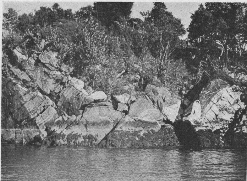
Fig. 3. Konkordante (til høyre) og transgressive pegmatittganger. (Concordant (right) and transgressive pegmatites.) Breivik, Gurskøy, T. Gjelsvik.
