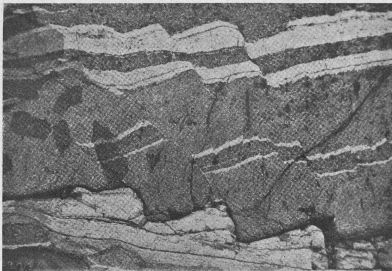
Fig. 15. Små forkastninger i båndet gneis. (Minor faults in banded gneiss.) Dryna, Vatne. Chr. C. Gleditsch.
