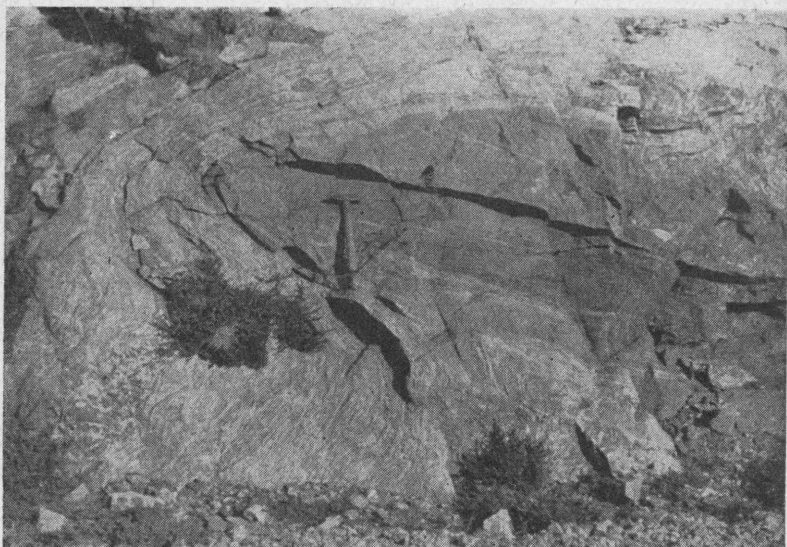
Fig. 11. Fold omkring basisk slire i gneisen. (Mafic lense inclosed in a fold in the coarsegrained gneiss.) Rjånes, Ørsta. Chr. C. Gleditsch.
