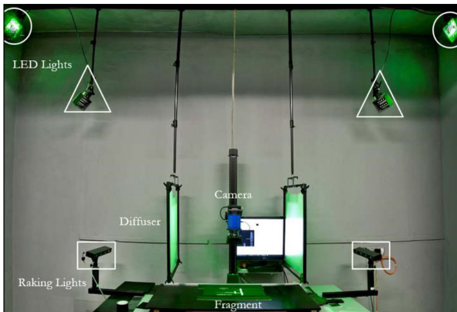
Fig. 5. MegaVision camera. Courtesy IAA. Credit: Shai Halevi.
