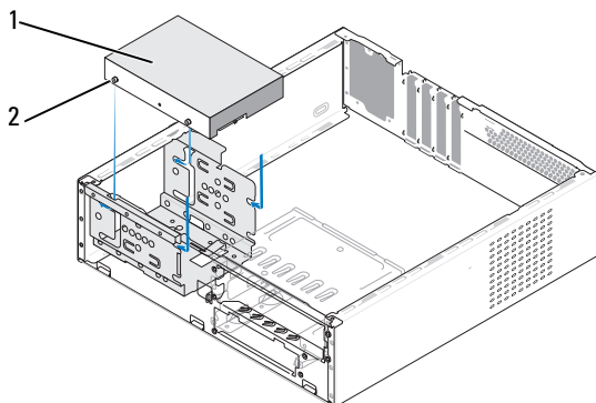
1 harddisk 2 skulderskruer (4)
