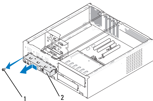
1 skruve 2 I/U-panel
