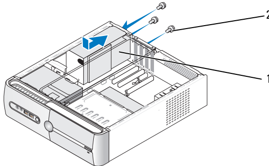
1 strømforsyning 2 skruer (3)
