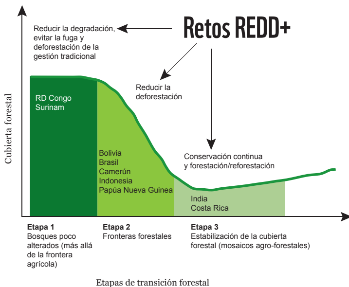
Figura 47. Modelo generalizado de transición forestal que destaca algunos de los desafíos asociados a REDD+ en diferentes países
