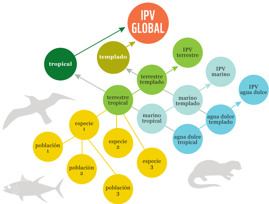
Figura 4. Configuración de los índices Planeta Vivo a partir de las tendencias poblacionales
