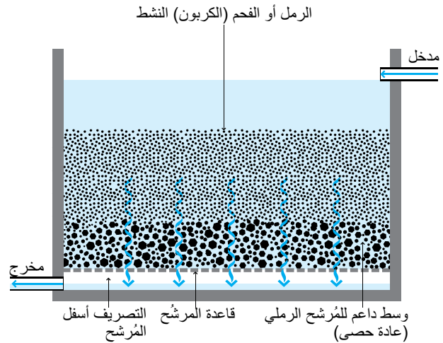
الترشيح الثلاثي (على سبيل المثال، الترشيح العميق)
