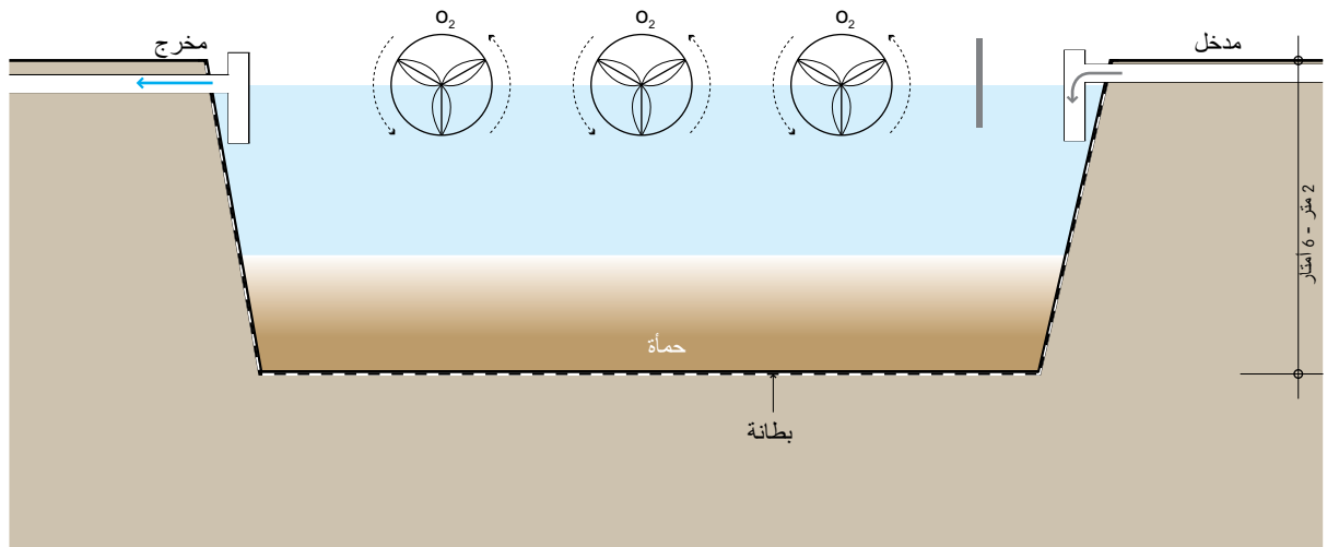
إمداد الأكسجين عن طريق مراوح التهوية
