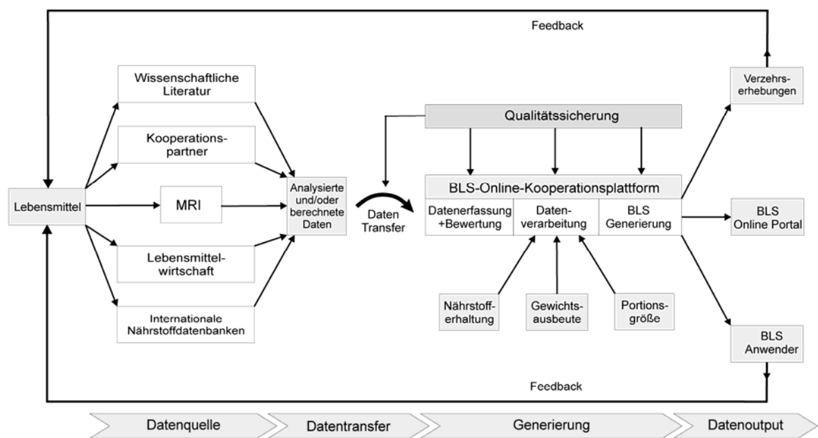
Abb. 3.1: BLS-Datenverarbeitung
