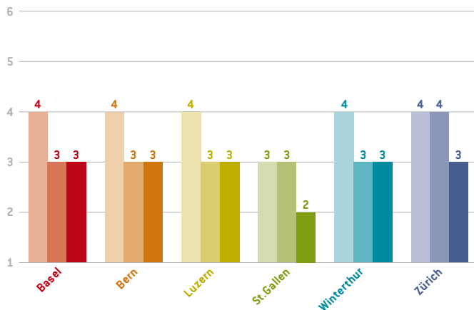
Abbildung 40: Luftschadstoffbelastung gemäss Langzeit-Belastungs-Index LBI Stand 2002, 2007 und 2013. 1 = geringe, 2 = mässige, 3 = deutliche, 4 = erhebliche, 5 = hohe, 6 = sehr hohe Belastung. ■ 2002 ■ 2007 ■ 2013
