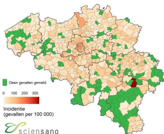
Verspreiding van de bevestigde gevallen per 100 000 inwoners tussen 21/8 en 3/9
